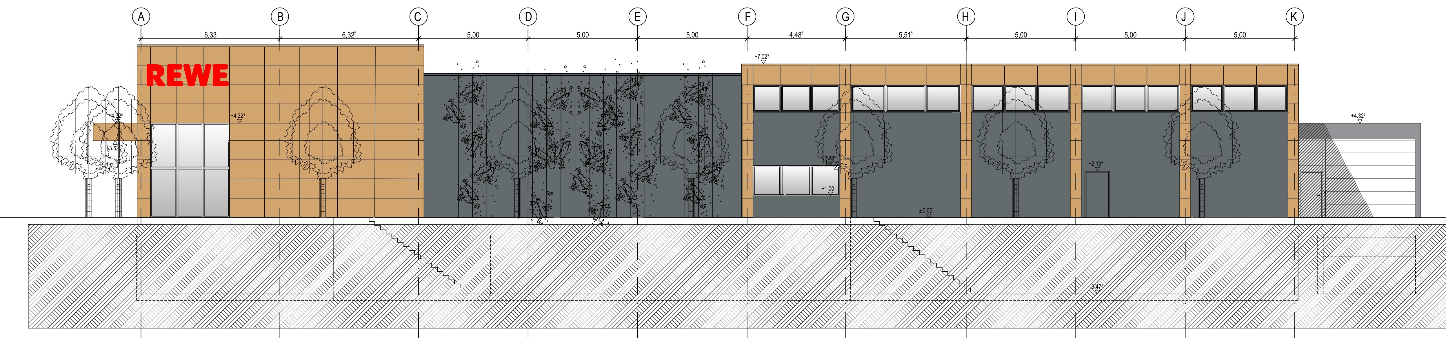
Nord - West Ansicht
