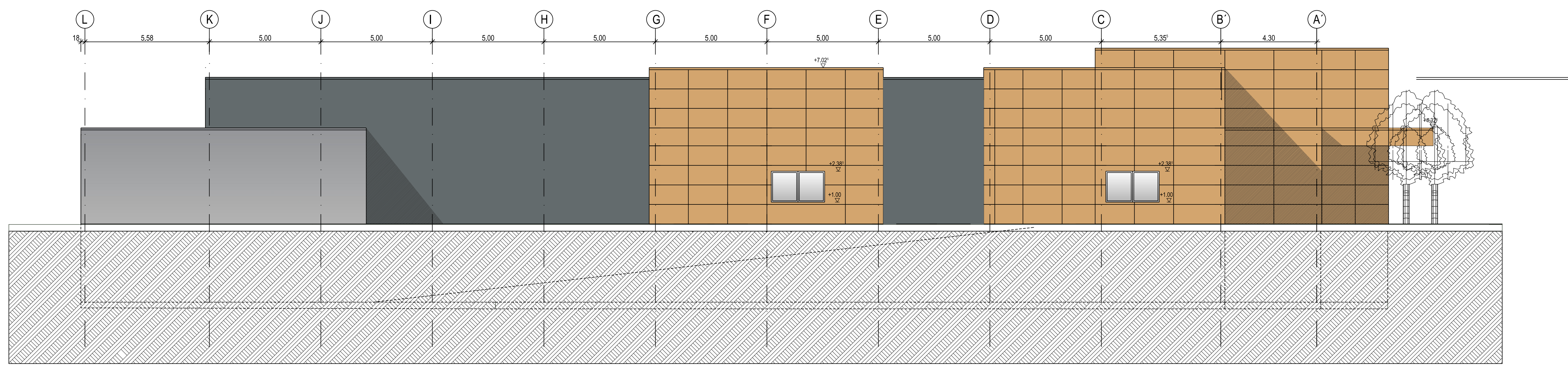
Süd - Ost Ansicht
