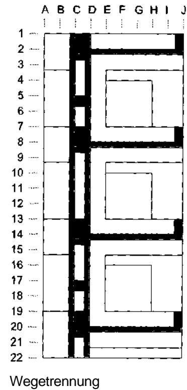
Hochbau-Typ 3 Kamm Ebene 03-06
