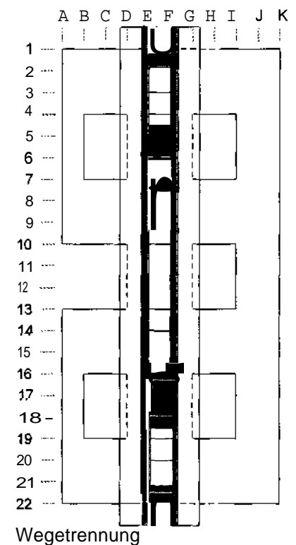
Hochbau-Typ 2 Riegel Ebene 03-06
