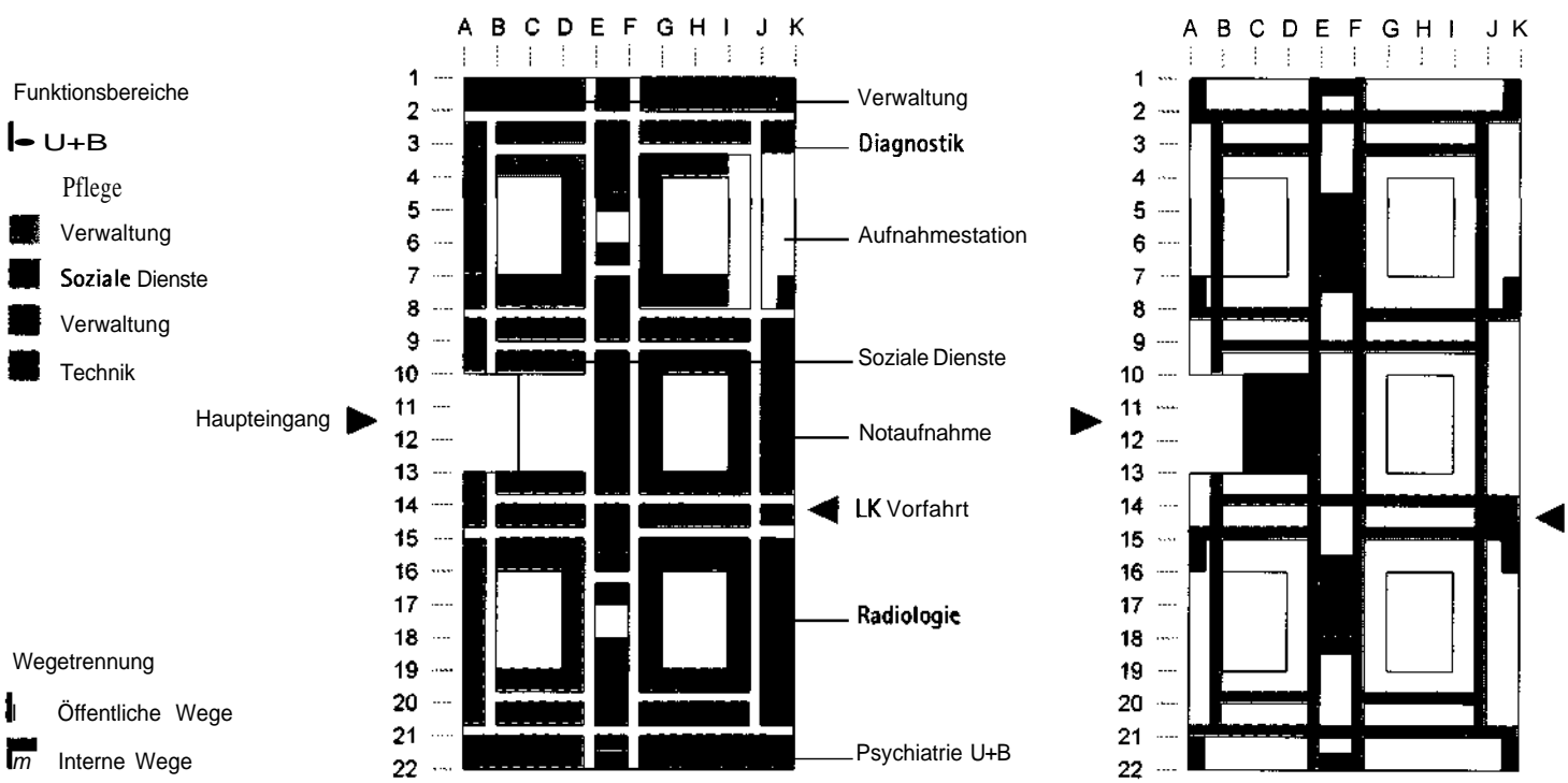
Hochbau-Typ 2 Riegel Ebene 00
