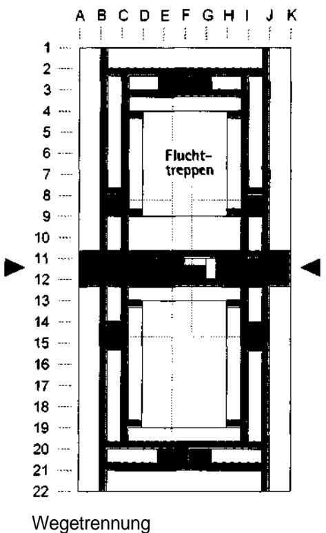
Hochbau-Typ 1 U Ebene 00
