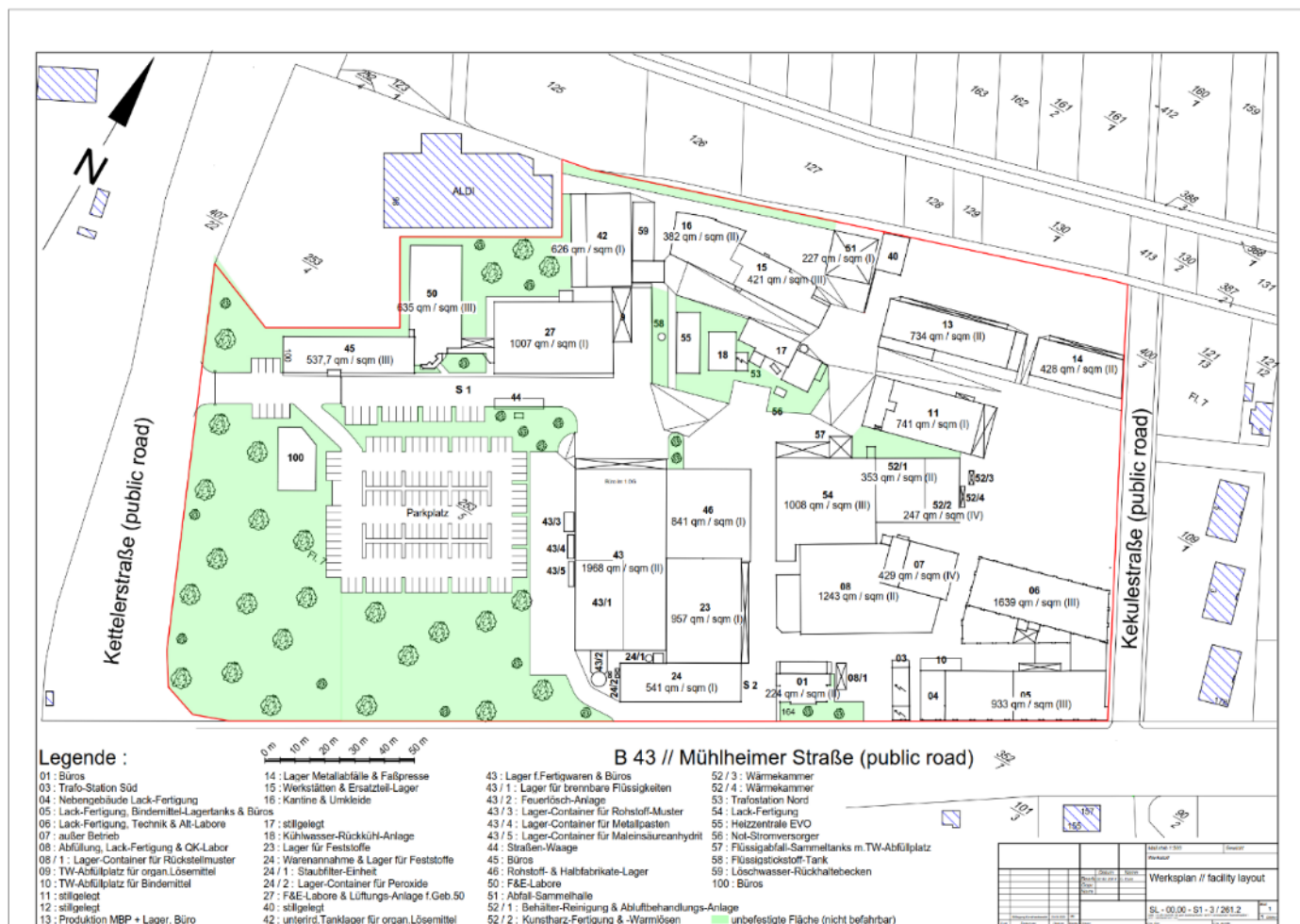
Abbildung 5: Werksplan der aktuellen Nutzung als Chemiefabrik zur Farbenherstellung
