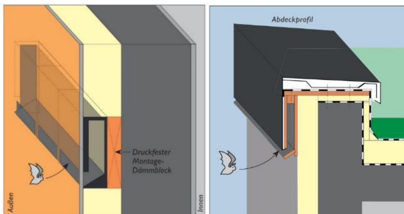
Abbildung 4: Beispiele künstlicher Fledermausquartiere. Einbaumöglichkeiten von Fledermausquartieren an Gebäuden (© Antje Schlameuß, Architektin)
