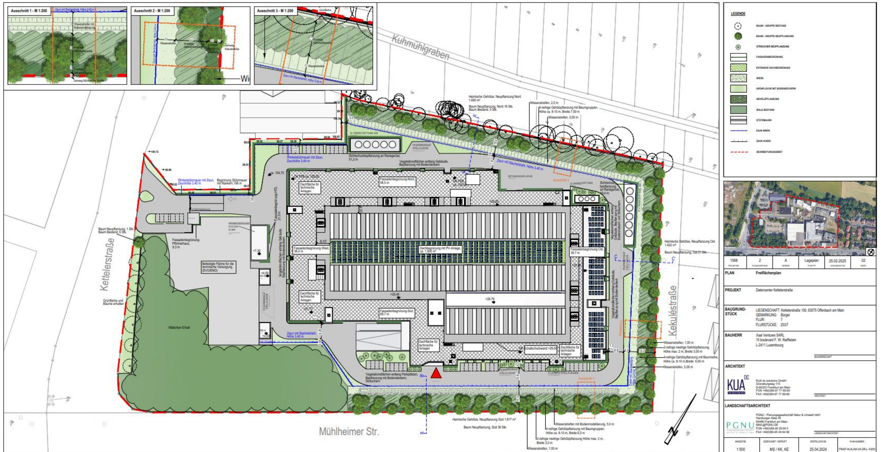
Abbildung 6: Planzeichnung des Vorhabens und vorgesehene Ausgestaltung der Freiflächen
