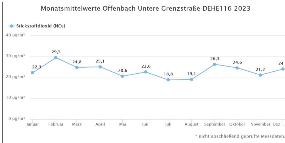
Abbildung 7: Stickstoffdioxid-Belastung in Offenbach im Jahr 2023
