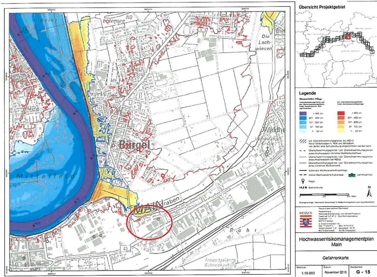
Abbildung 3: Plan Hochwasserrisikomanagement
