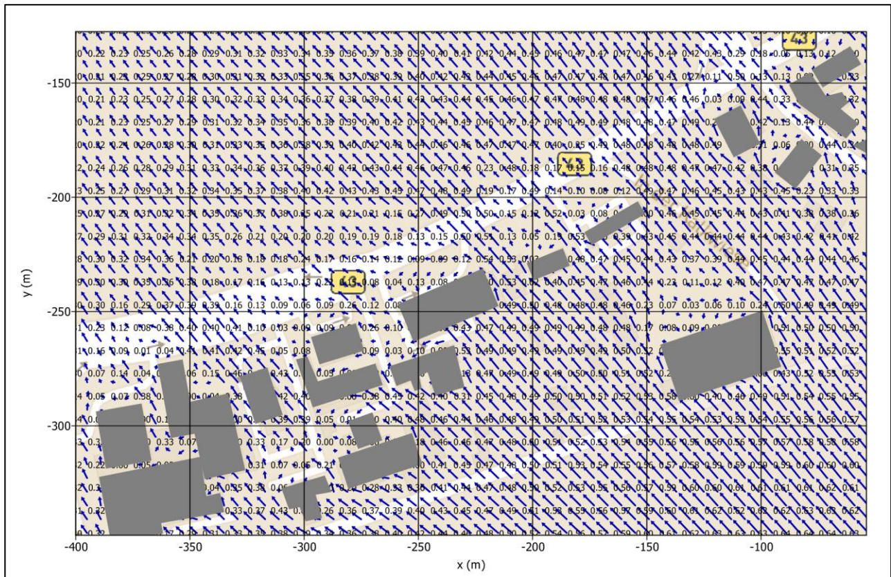
Abbildung 21: Kaltluftströmung am Beurteilungspunkt Mühlheimer Straße im gegenwärtigen Zustand (Variante 1)
