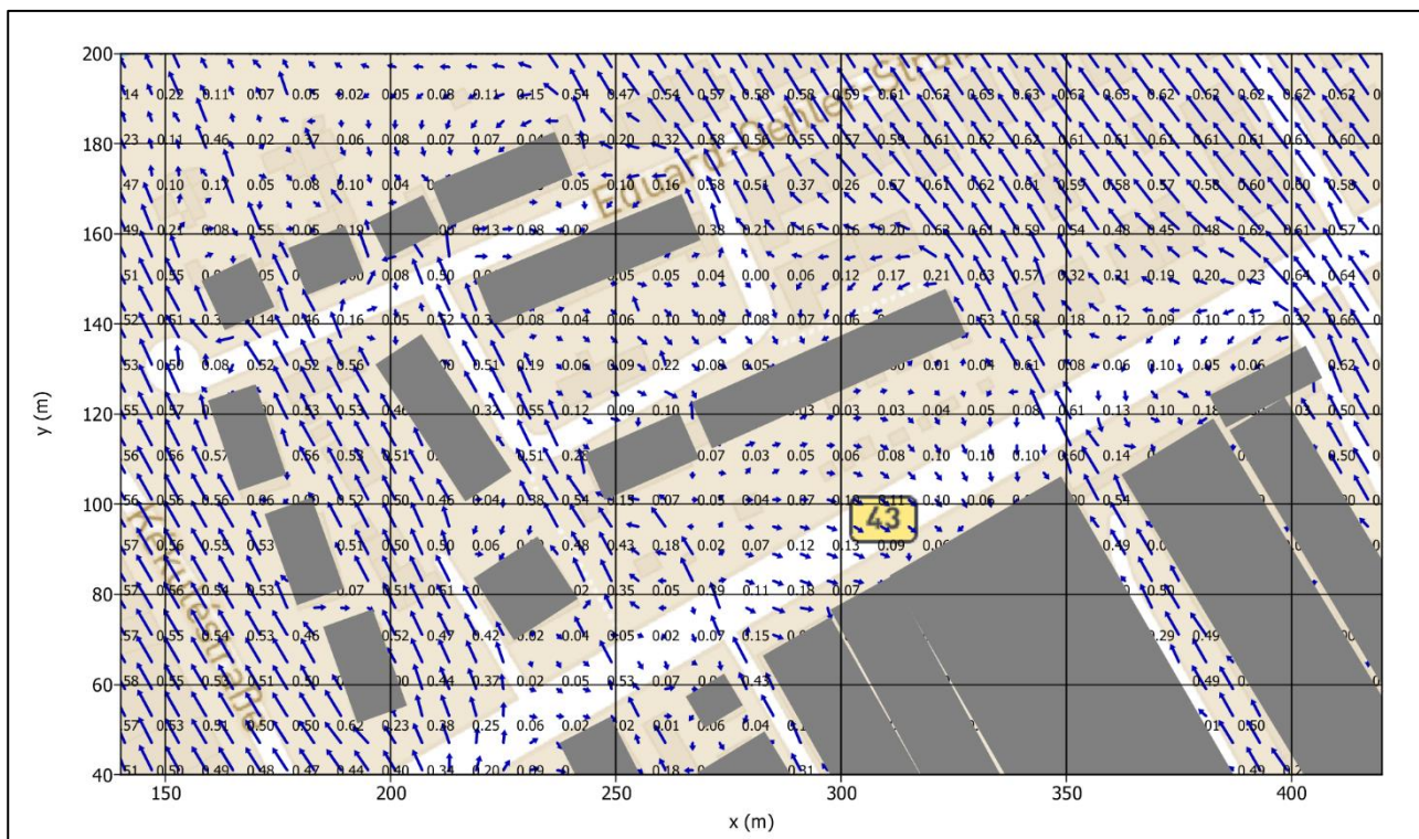
Abbildung 20: Kaltluftströmung am Beurteilungspunkt Kekulestraße mit geplanter Wärmeemission (Variante 3)
